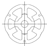
明和標準6-4極SRMコア
