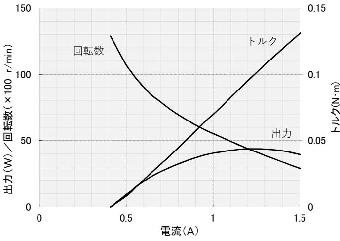
UM-M5モーター-G03 特性
