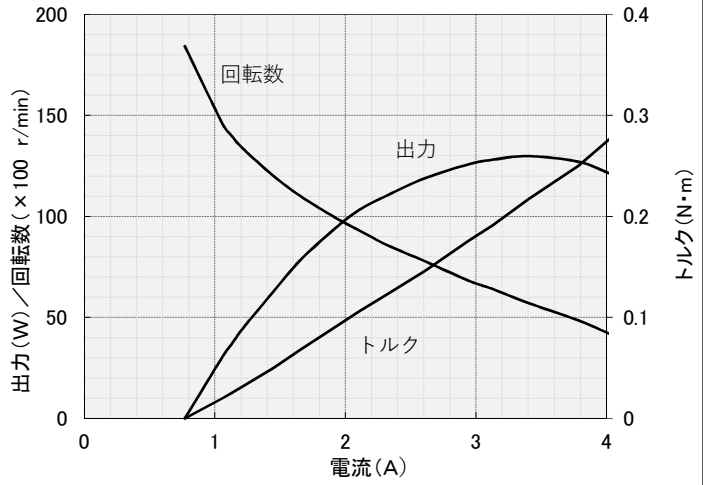
UM-M5モーター-G02 特性
